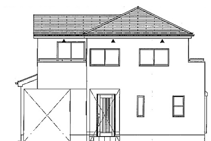
西立面図
